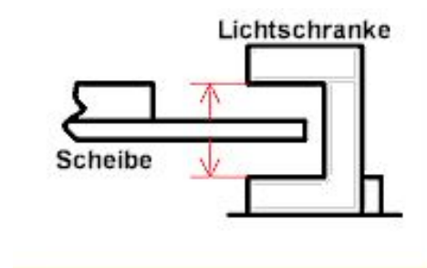
Abbildung 3 Ausrichtung von Sektorscheibe und Lichtschranke.
