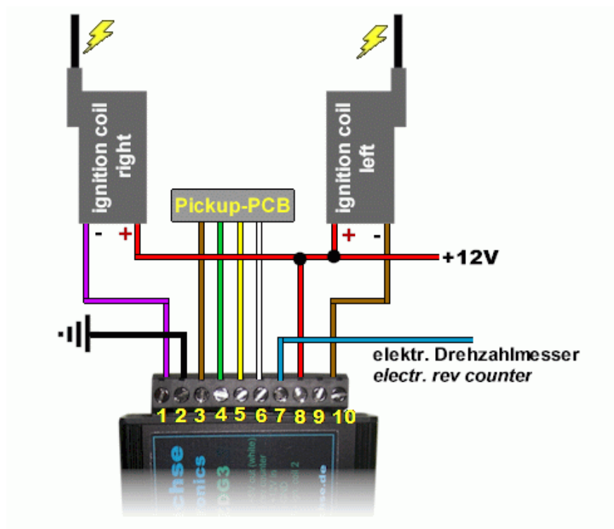
Elektrischer Anschluss der Zündung mit zwei 12V-Zündspulen.
