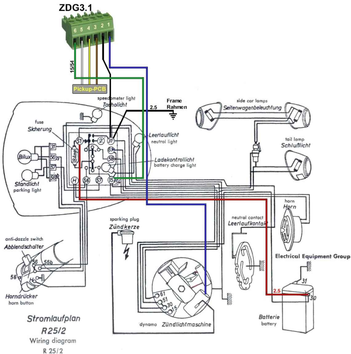
Anschlussschema
