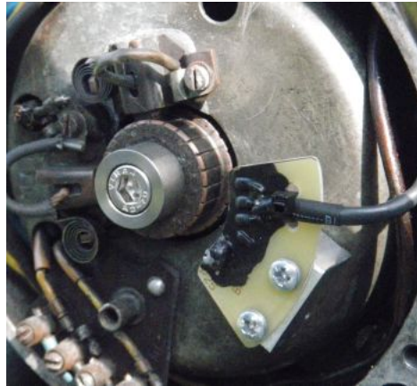
Die Rotormittelschraube entfernen und durch die mitgelieferte Inbusschraube und dem Mitnehmer ersetzen. Zuletzt wird der Magnetring auf den Mitnehmer aufgeschoben, aber die Madenschrauben noch nicht festziehen.
