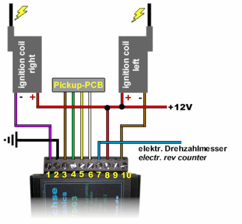
Abbildung 4 Anschluß mit zwei Einzelspulen (ZDG 3.23).
