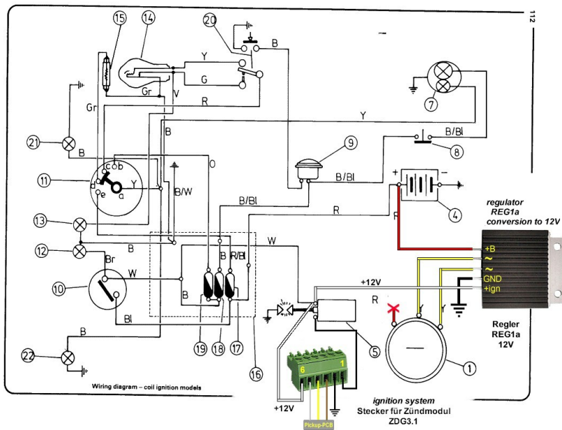
Elektrischer Anschluss der Zündung
