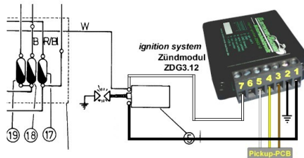
Anschluss im Stromlaufplan
