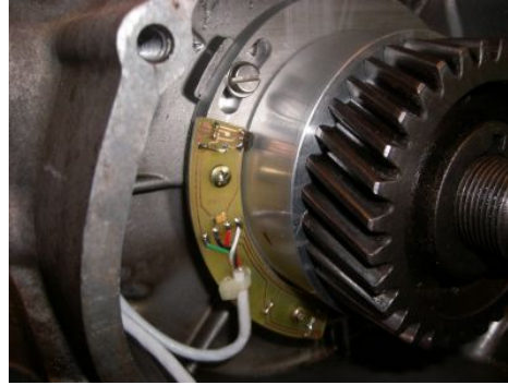
Befestigung des neuen Magnetringes am Primärzahnrad.
