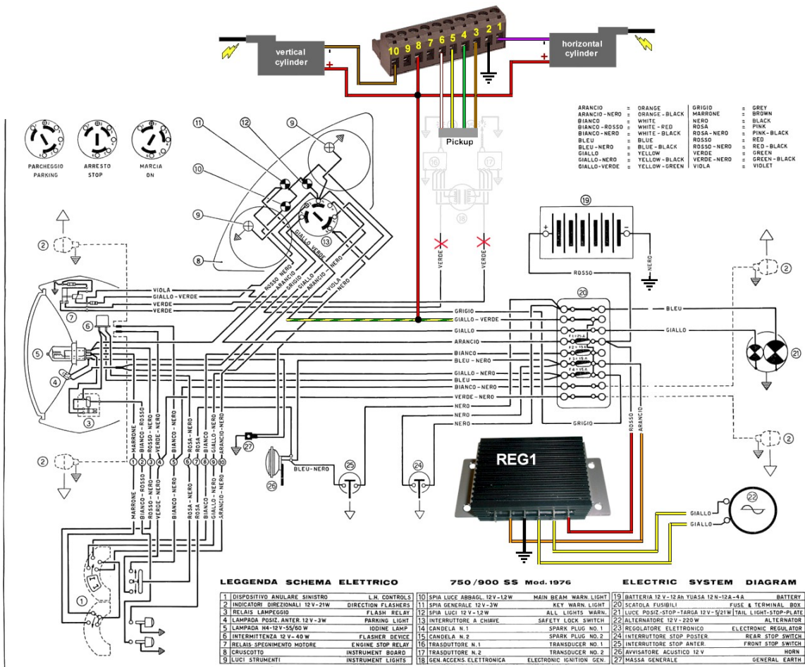
Komplette Ansicht des Stromlaufplans
