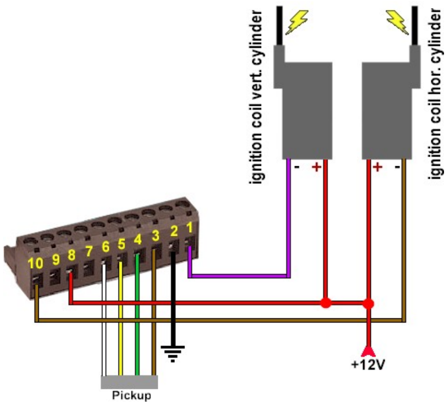
Abbildung 3 Anschlußschema
