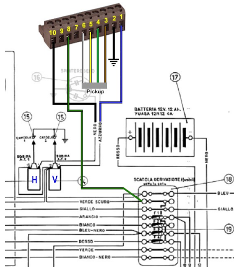
Abbildung 4 Anschluß im Stromlaufplan.
