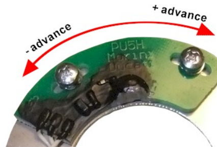
Abbildung 7 Feineinstellung des Versatzes der Frühzündung zwischen den beiden Zylindern.
