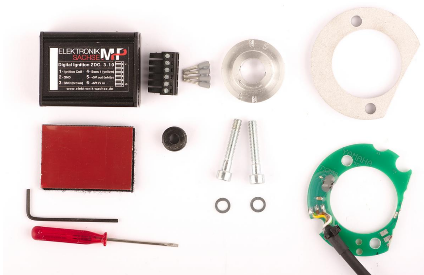
Abbildung 1 Lieferumfang
