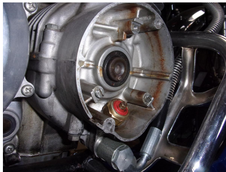
Abbildung 2 Entfernen der übrigen Komponenten der alten Zündung.
