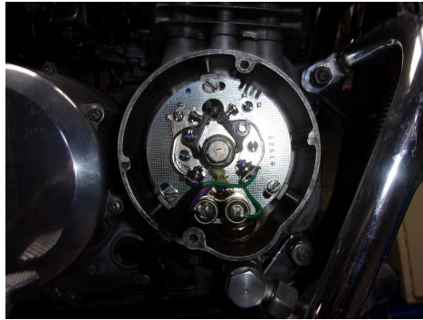
Abbildung 2 Die alten Zündungskomponenten werden entfernt
