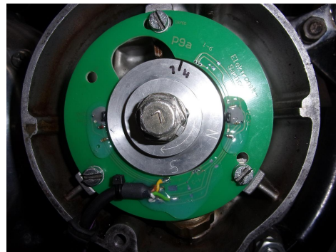
Abbildung 2 Montage des neuen Pickups, Mitnehmers und des Magnetrings. Die Madenschrauben im Magnetring noch nicht anziehen.
