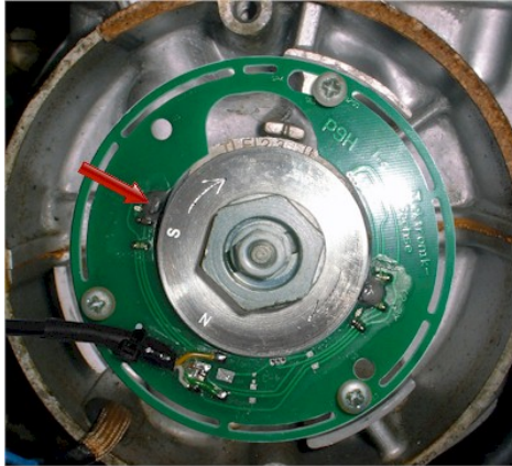
Abbildung 7 Dieser Sensor wird für die Grundeinstellung verwendet.
