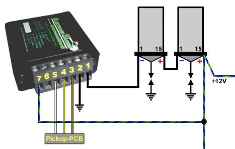
Anschlußdiagramm mit zwei 6 V-Spulen in Reihe.
