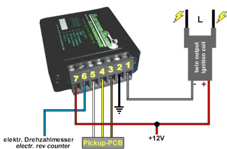
Anschlußdiagramm mit einer 12 V-Doppelzündspule.
