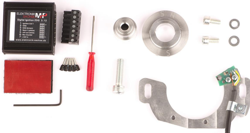
Abbildung 1 Lieferumfang
