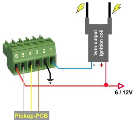
Anschlußdiagramm mit einer 6 V-Doppelzündspule.
