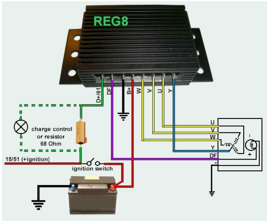
Abbildung 1 Schematische Darstellung des Regleranschlusses
