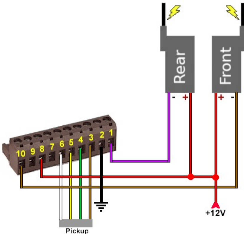
Anschlussplan
