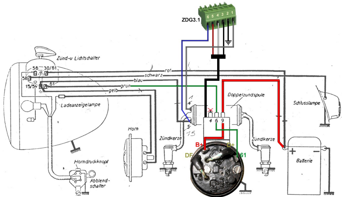
Anschluss im Schaltbild
