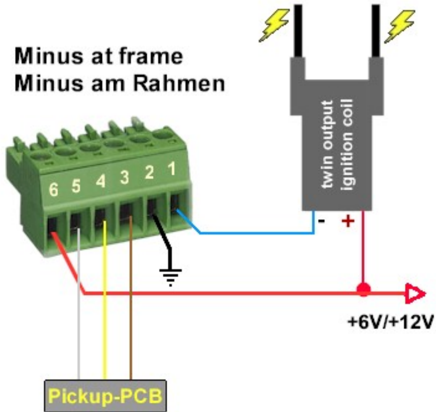
Anschlusschema
