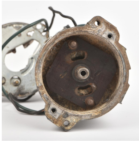
Abbildung 3 Der leere Verteiler.
