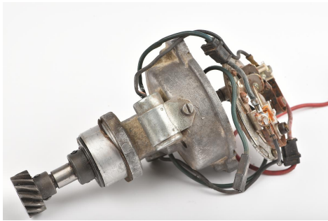
Abbildung 2 Entfernen der Kontakte aus dem Verteiler.
