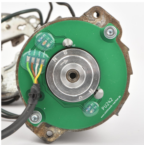
Abbildung 6 Montage der Magnetringes.
