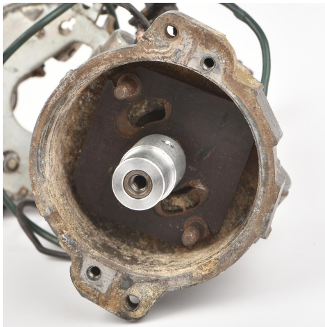
Abbildung 4 Montage des Mitnehmers.
