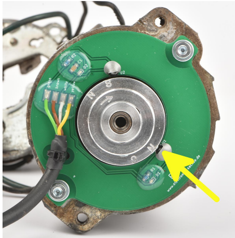
Abbildung 10 Der Sensor der für die Grundeinstellung verwendet wird.
