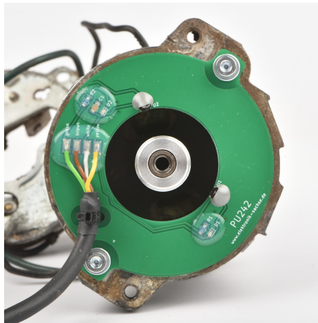
Abbildung 5 Montage des Pickups.
