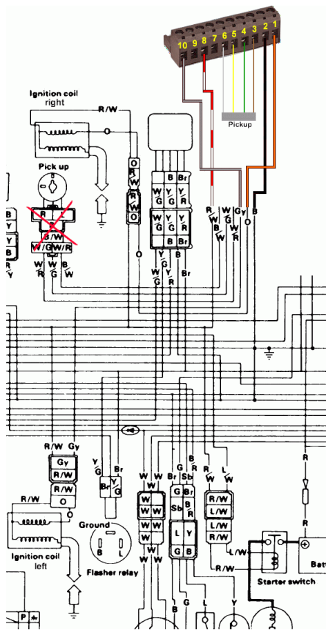
Anschlusschema am '81er Modell
