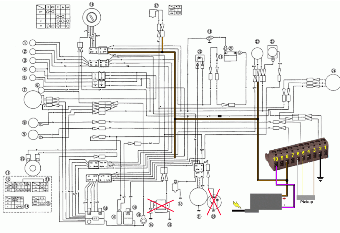
Anschlusschema
