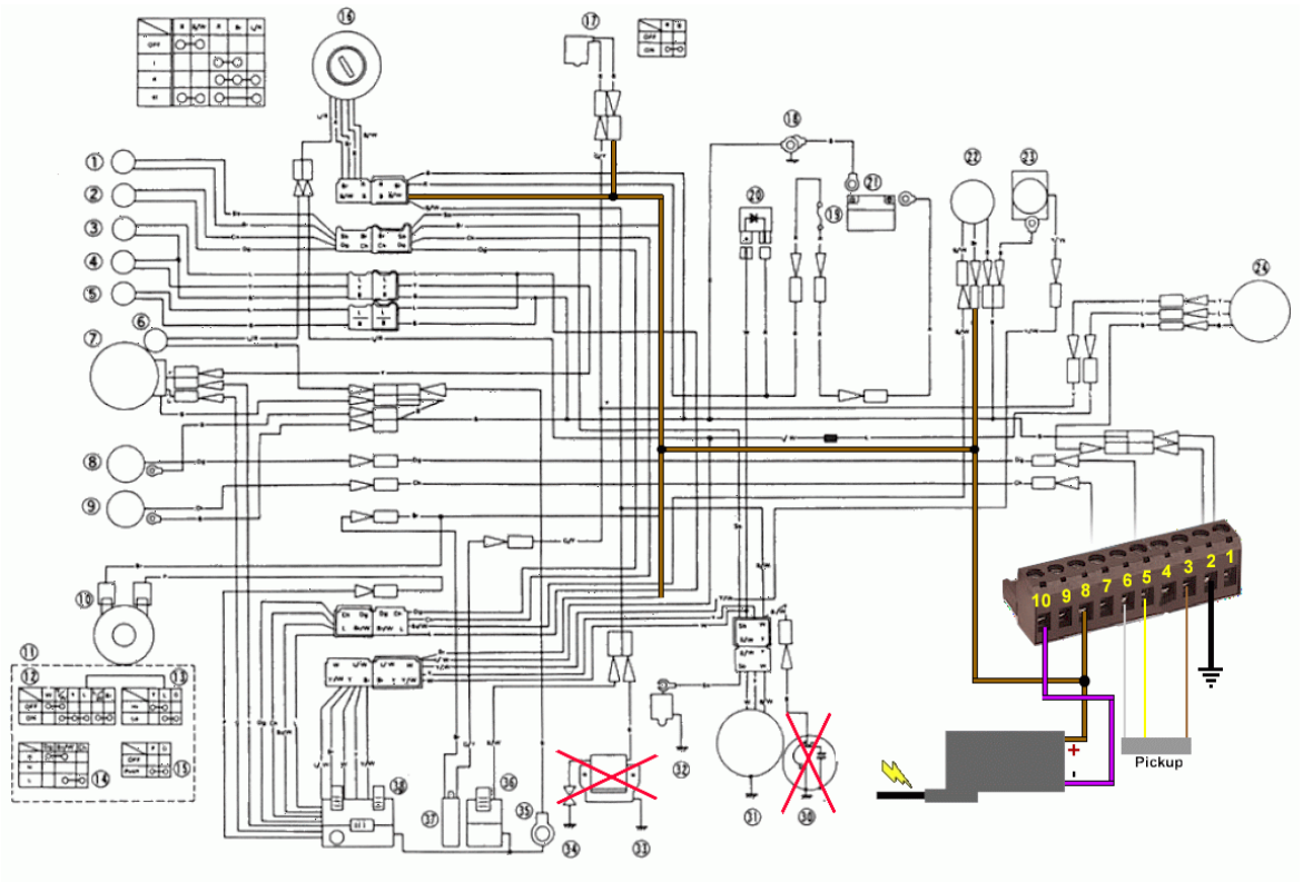
Anschlusschema
