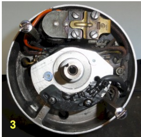
Abbildung 2 Montage des neuen Pickups.
