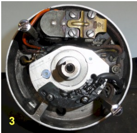
Abbildung 2.d Montage des neuen Pickups.
