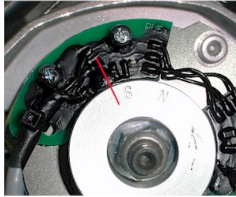
Abbildung 6.b Dieser Sensor wird für die Grundeinstellung benutzt.
