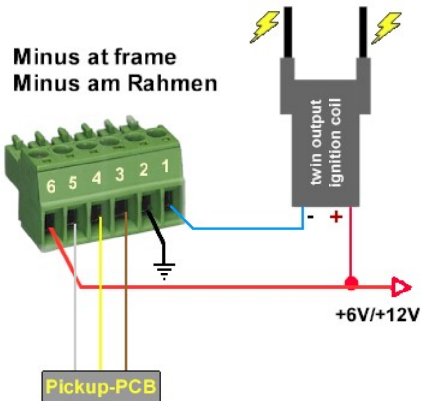
Anschlussplan Elektronik 3.10
