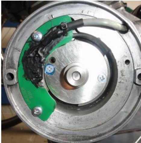
Abbildung 2.d Montage des Pickups.
