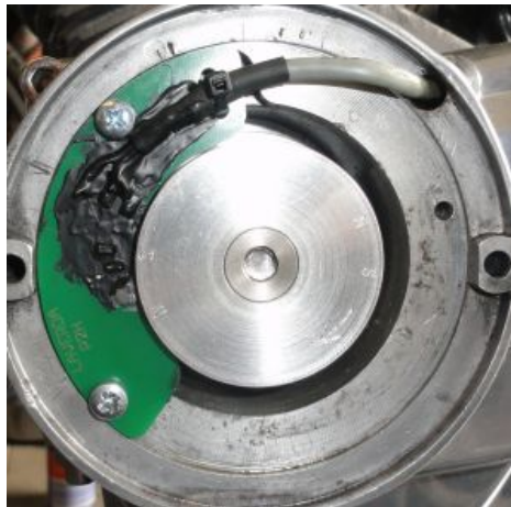
Abbildung 2.e Montage des Magnetrings.
