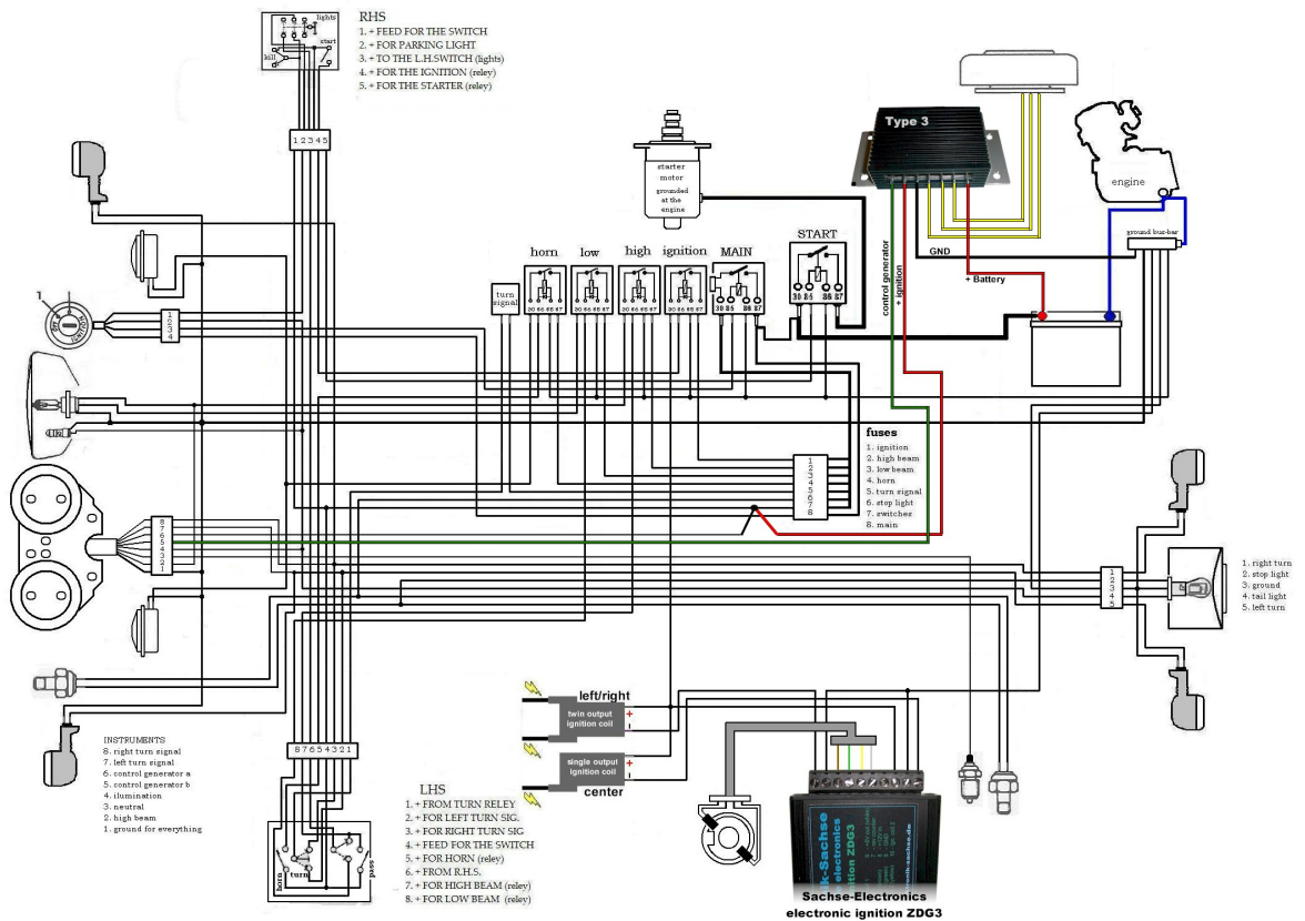
Abbildung 4 Anschluß im Stromlaufplan.
