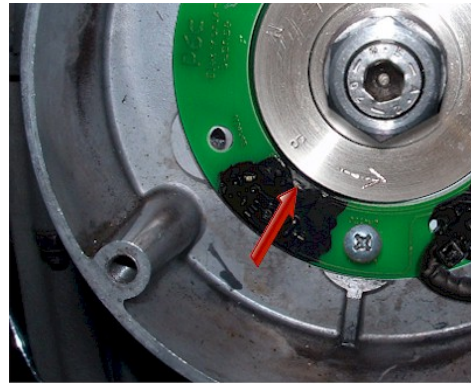
Abbildung 7.b Die LED geht aus wenn der Kolben auf OT ist.
