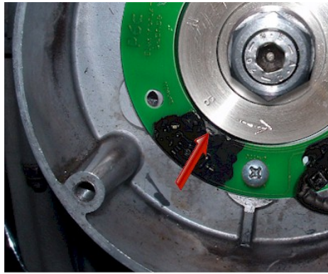
Abbildung 7 Die LED geht aus wenn der Kolben auf OT ist.
