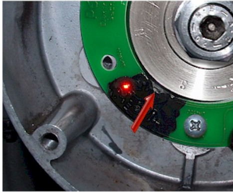
Abbildung 7 Dieser Sensor wird für die Grundeinstellung benutzt.
