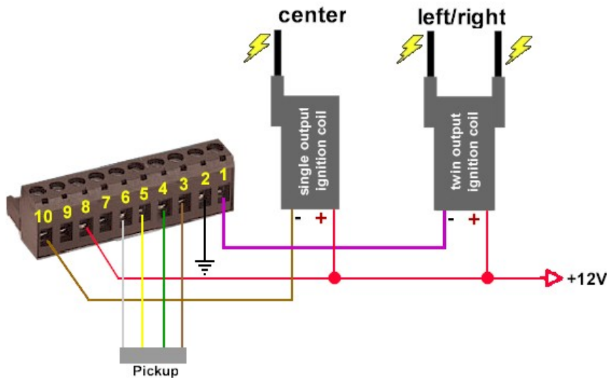
Abbildung 3 Elektrischer Anschluß der Zündung.
