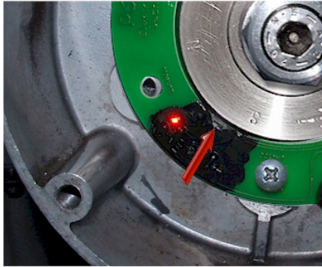
Abbildung 7.a Dieser Sensor wird für die Grundeinstellung benutzt.
