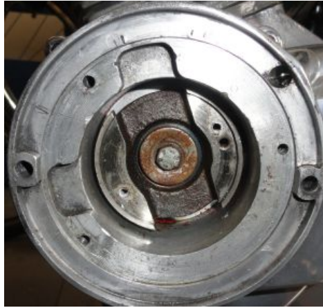
Abbildung 2.a Entfernen der alten Komponenten.
