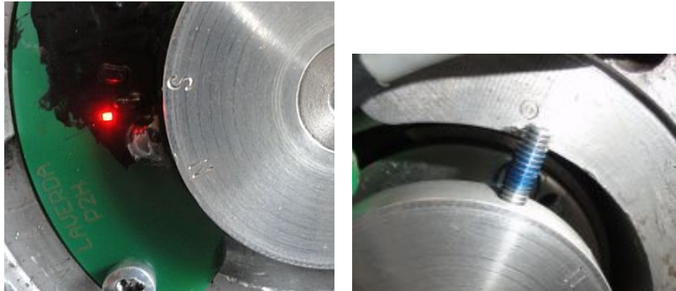
Abbildung 7 Einstellung und Montage des Magnetrings
