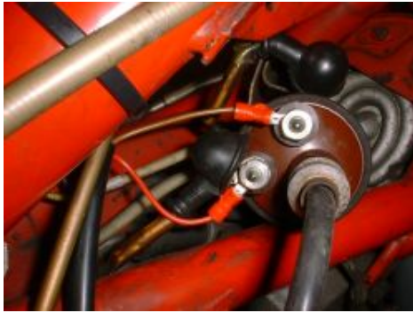
Abbildung 3 Montagevorschlag der rechten Zündspule.
