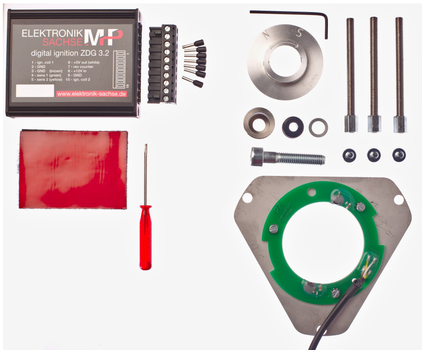
Abbildung 1 Lieferumfang
