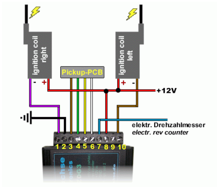
Abbildung 6 Anschlußschema
