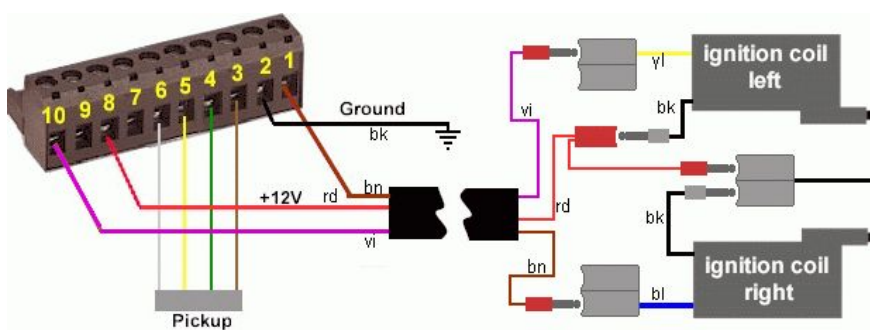
Elektrischer Anschluss der Zündung
