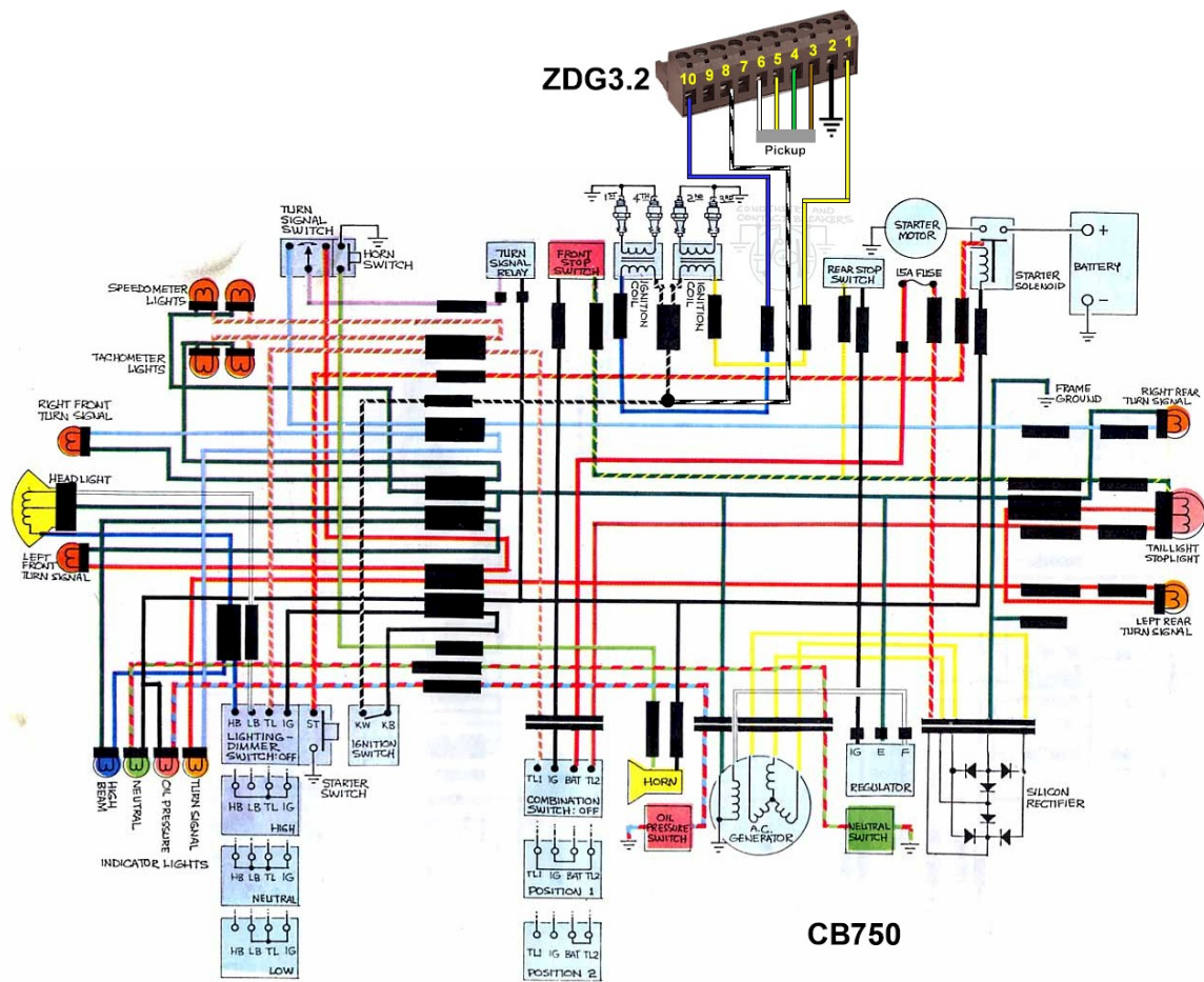
Abbildung 5 Anschluß im Stromlaufplan.
