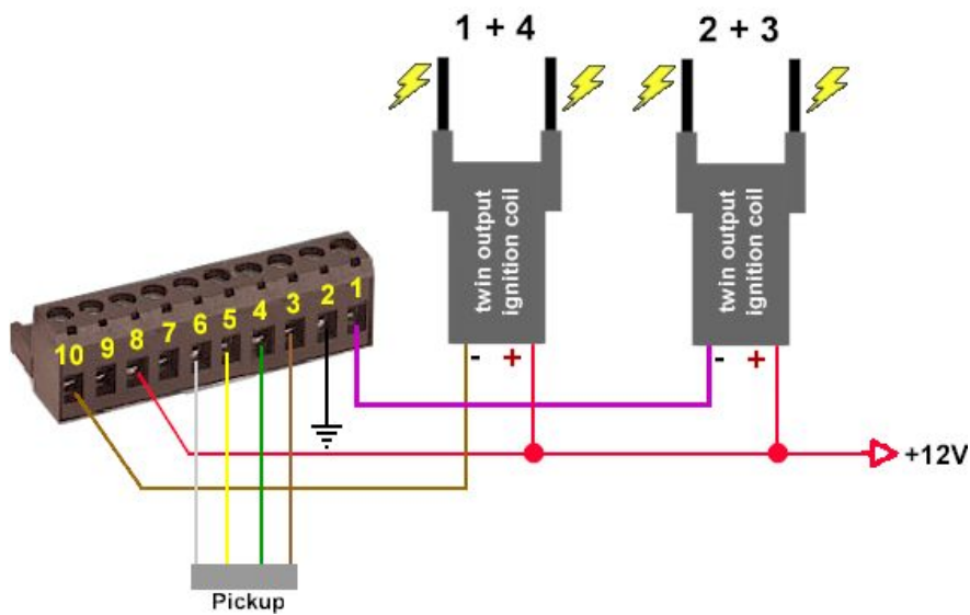
Abbildung 4 Elektrischer Anschluss der Zündung.
