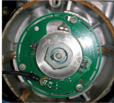
Abbildung 3 Fertige Montage des Pickups und unseres Mitnehmers.
