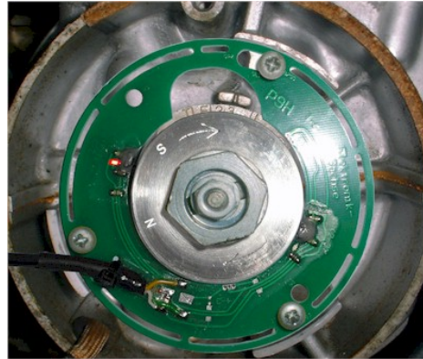
Abbildung 8.b Die LED geht an, wenn der S-Magnet am Sensor vorbeiläuft.
