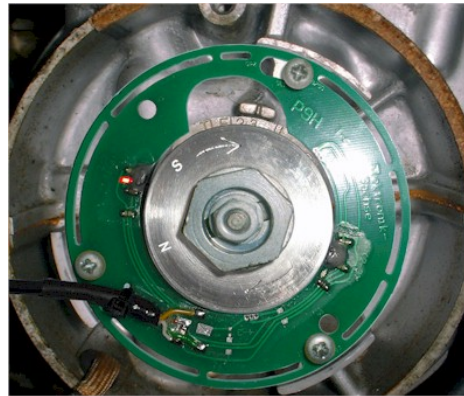
Abbildung 8 Die LED geht an, wenn der S-Magnet am Sensor vorbeiläuft.
