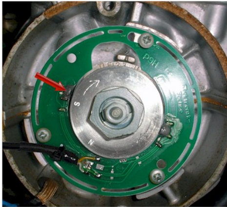
Abbildung 8 Auf diesem Sensor wird die Grundeinstellung gemacht.
