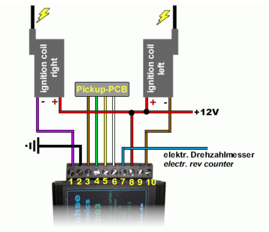
Abbildung 3 Anschlußschema
