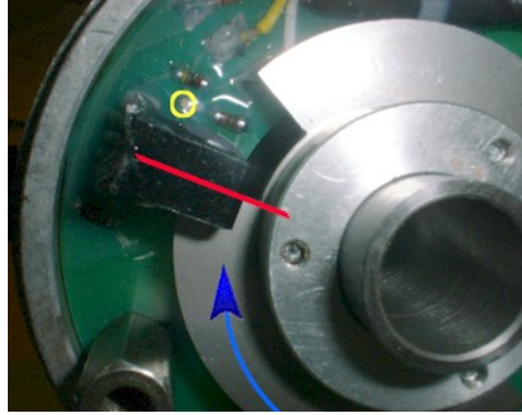
Abbildung 6 Wenn die LED auf OT ausgeht, dann ist die Zündung korrekt eingestellt. Zu beachten ist, daß diese Abbildung die ältere optische Version zeigt.
