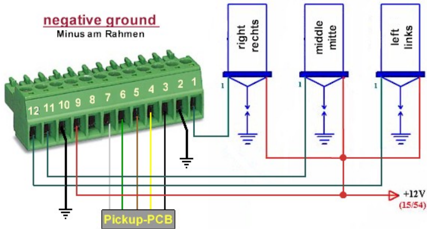
Anschlussschema der Zündung mit Minus am Rahmen
