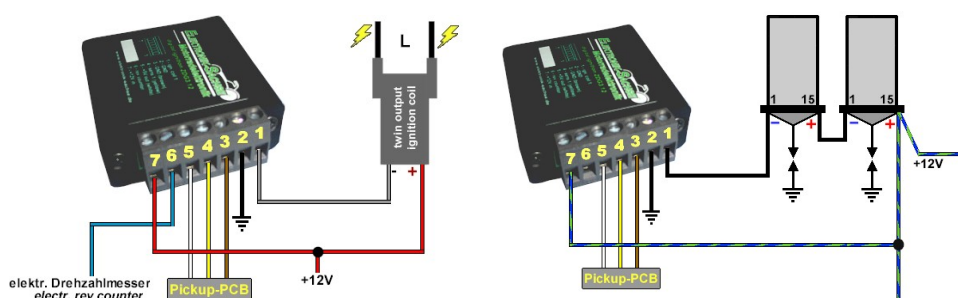
Elektrischer Anschluss der Zündung mit einer 12 V-Doppelzündspule.
